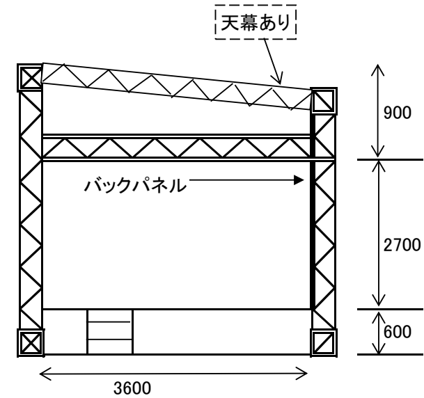
側面図
